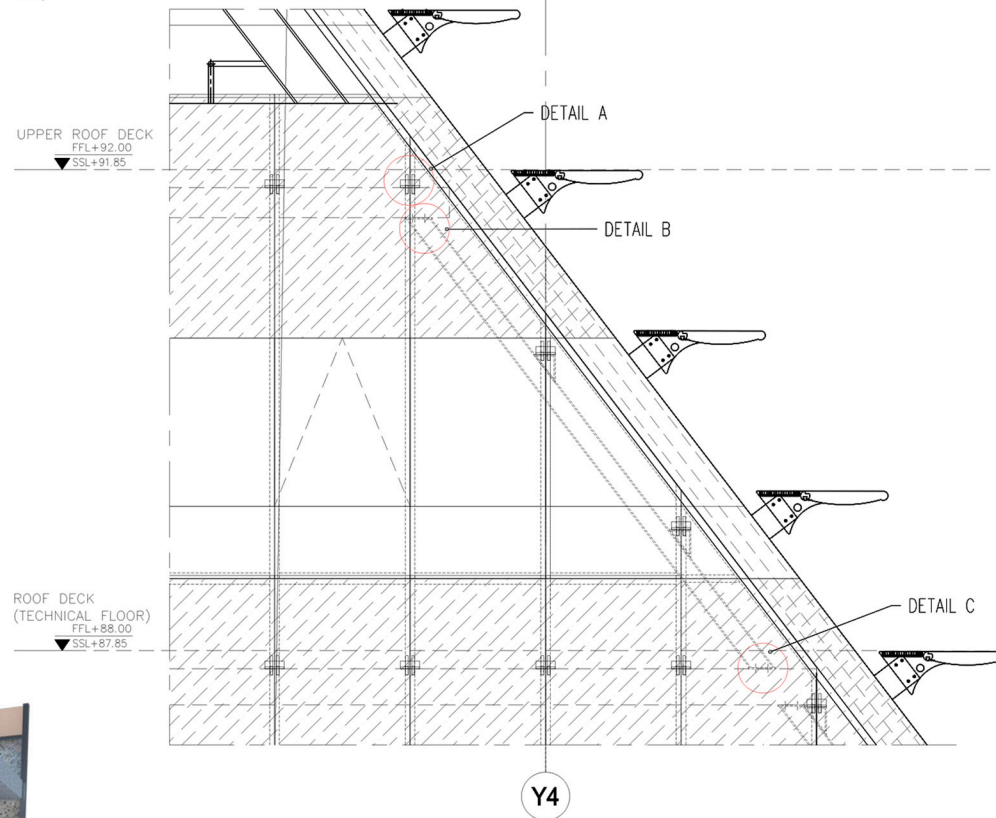
ELEVATION 1:20
