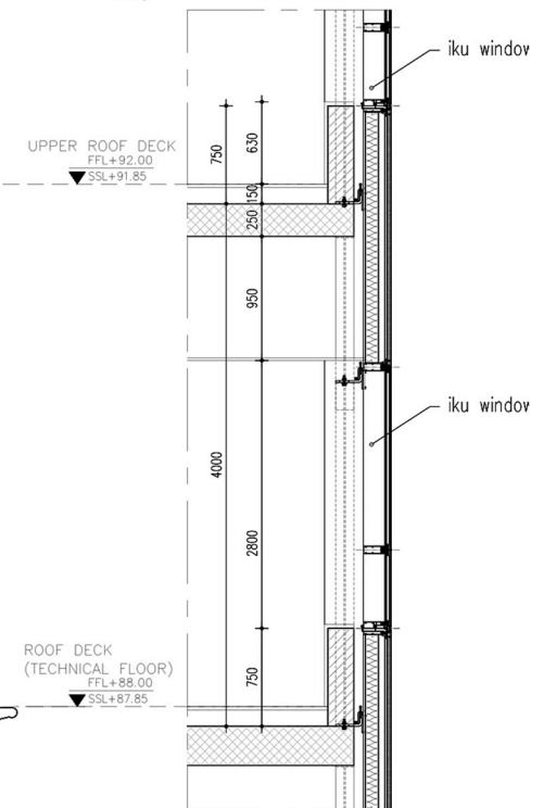
SECTION 1-1 1:20
