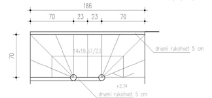
osnova sprata r 1:20
