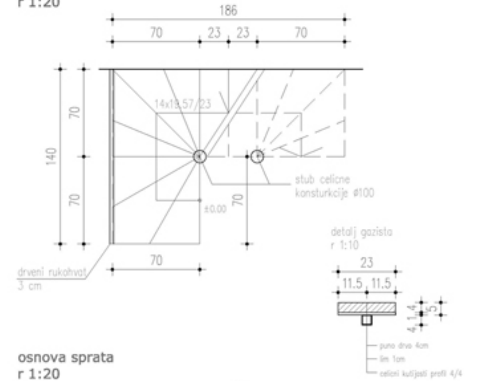
osnova prizemlja r 1:20
