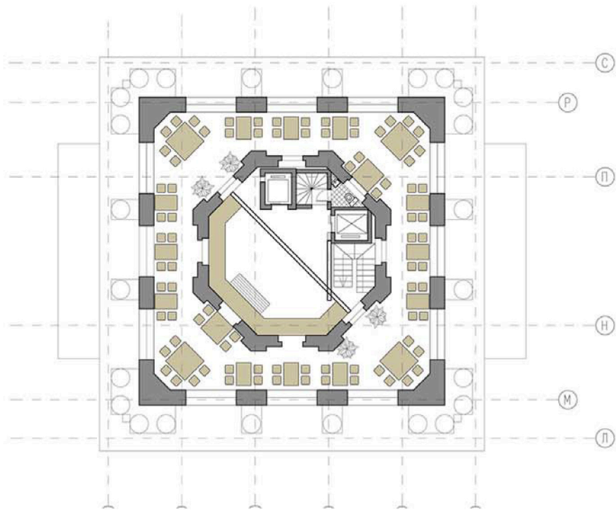
план 31.-го этажа +116.43
